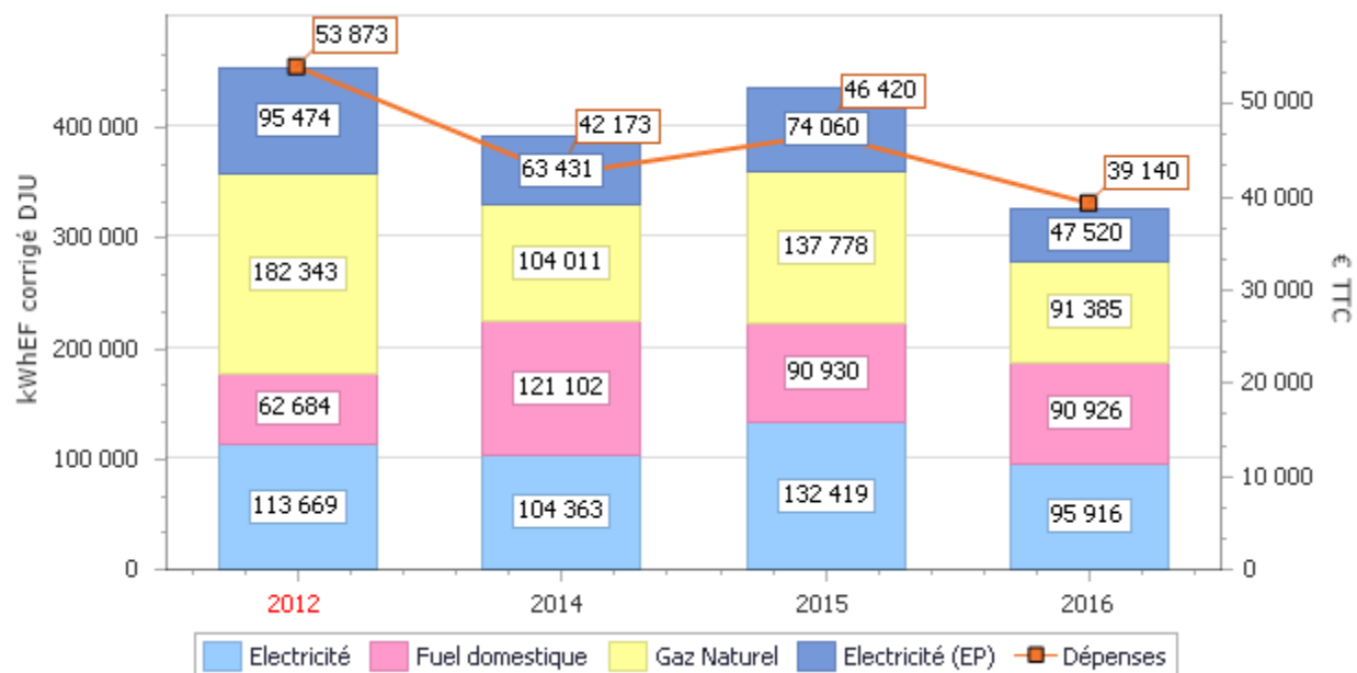
Figure 1 : Consommations d'énergie corrigées DJU et dépenses
