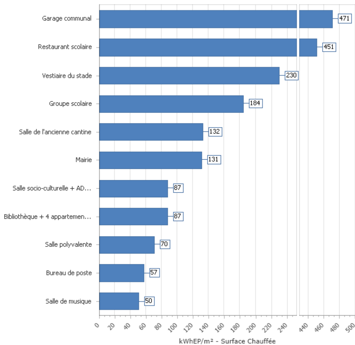
Figure 24 : Classement des établissements suivant la performance énergétique (2016)
