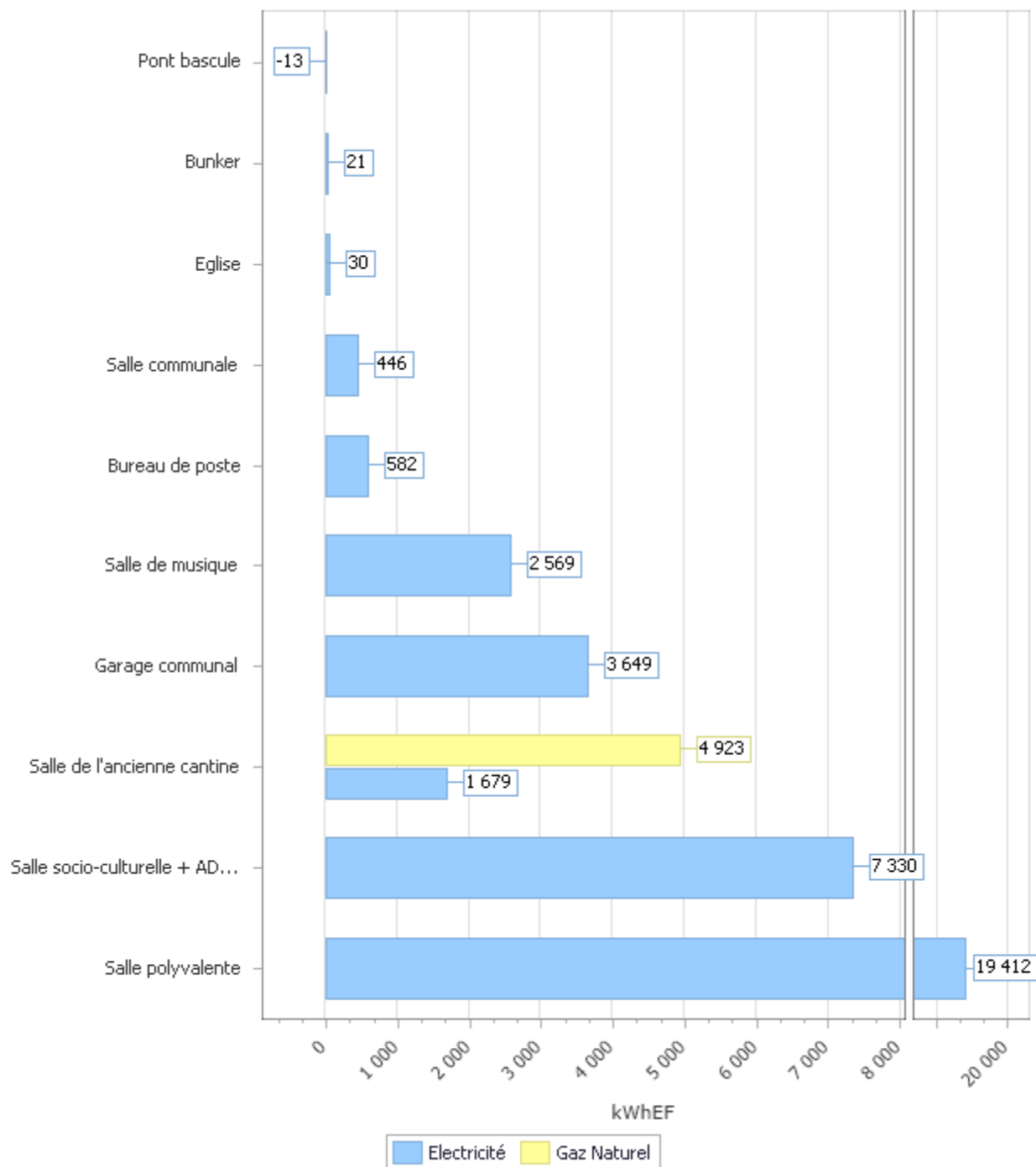
Figure 18 : Consommations par énergie et par établissement (2016) (Top 1 à 10)
