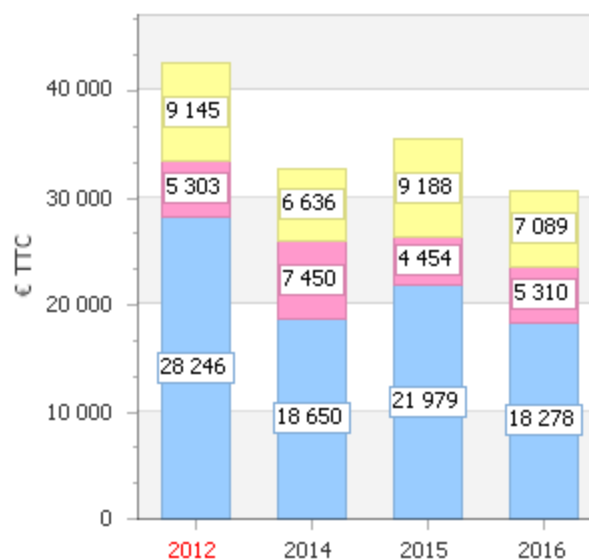
Figure 4 : Evolution des consommations corrigées DJU par énergie
