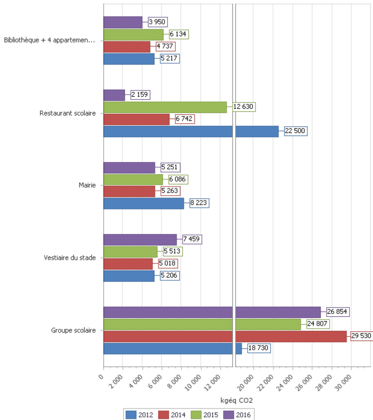
Figure 14 : Evolution des émissions de GES par établissement (Top 11 à 15)
