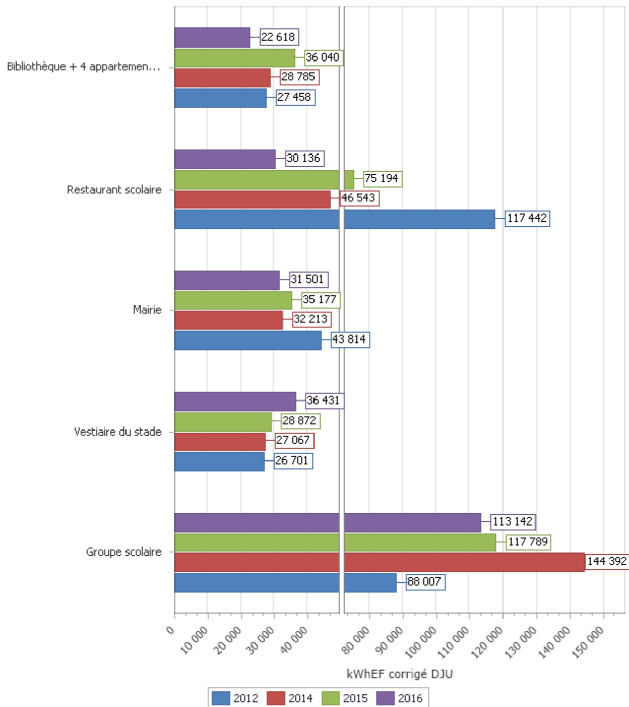
Figure 10 : Evolution des consommations corrigées DJU par établissement (Top 11 à 15)
