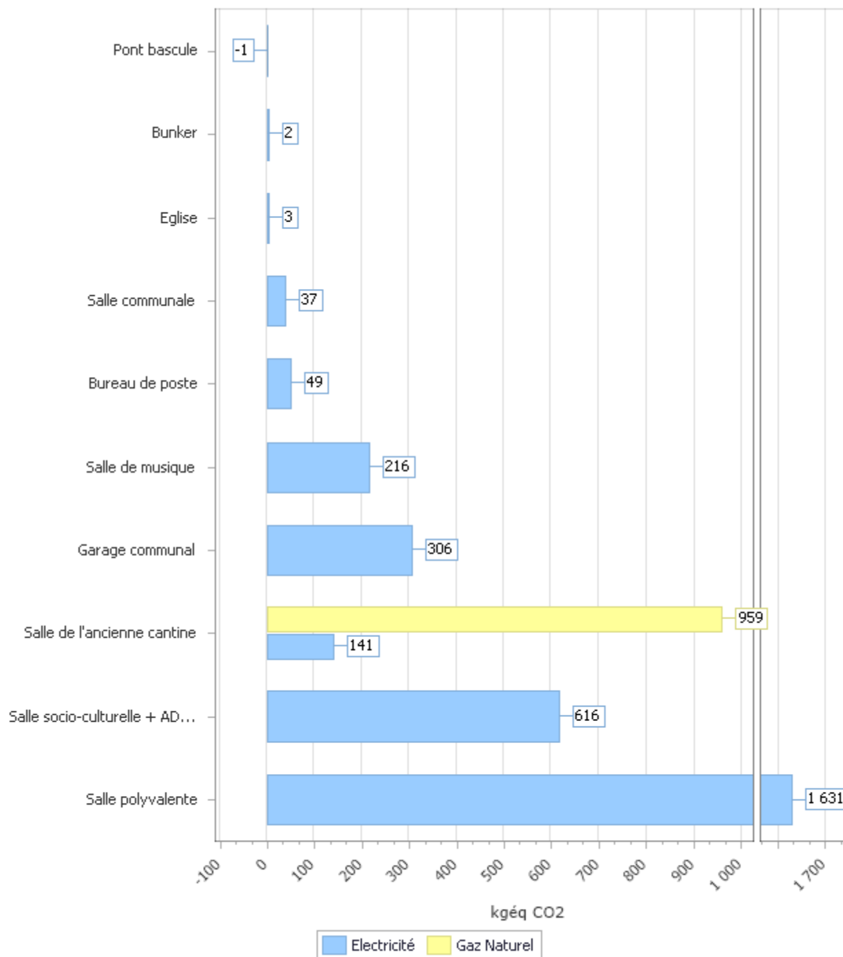
Figure 22 : Emissions de GES par énergie et par établissement (2016) (Top 1 à 10)
