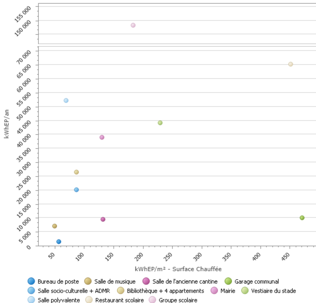
Figure 25 : Classement des établissements par performance énergétique et consommation (2016)
